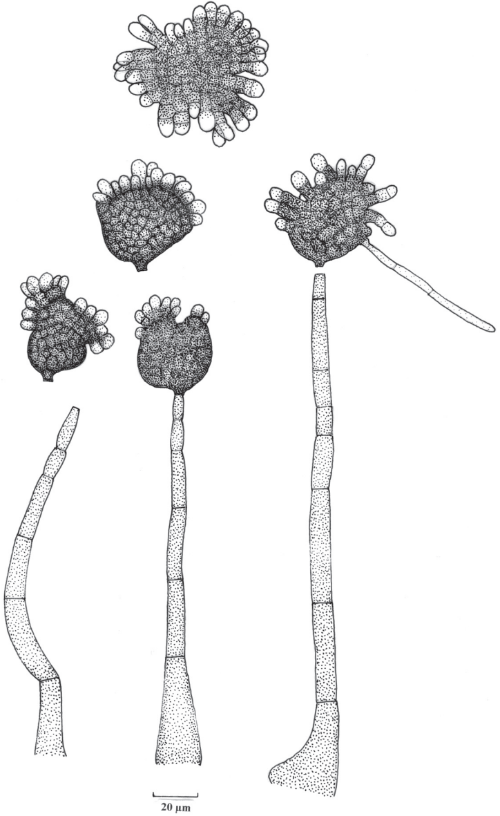
FIG. 1. Digitoramispora tambdisurlensis . Conidiophores and conidia.
